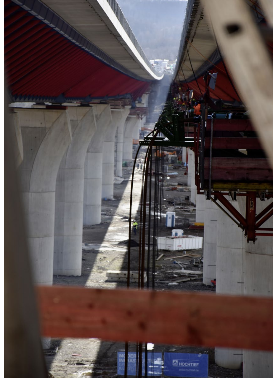
Der Überbau hat sein Ziel auf den neuen Pfeilern fast erreicht. Die Hydraulikaggregate waren seitlich an diesen Pfeilern angesetzt.
