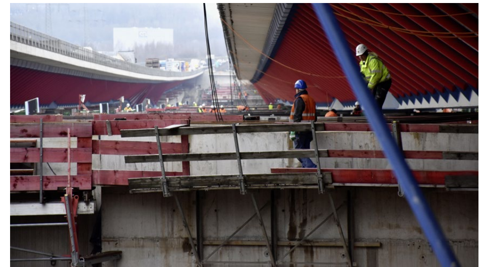
Auf jedem der 13 Pfeiler überwachten Techniker minutiös den Verschub.
